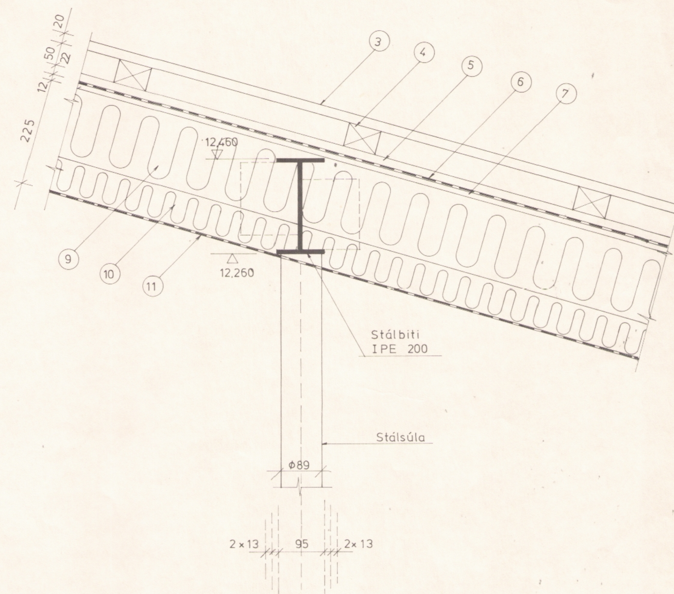
20 108 Snid í þak við stálbita 1:5
