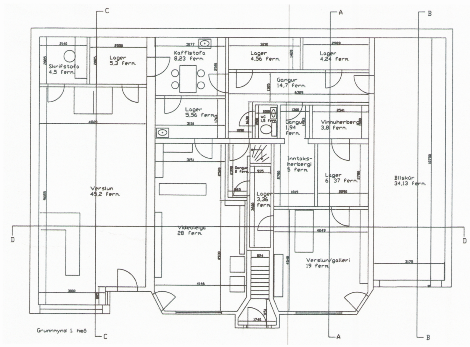
Grunnmynd 1. hæð 1 : 100
