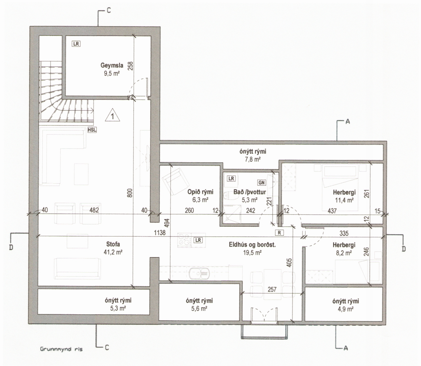
Grunnmynd ris 1 : 100
