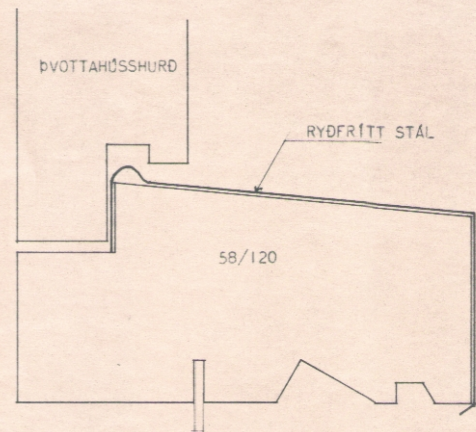
UNDIRSTYKKI MED HURÐ
