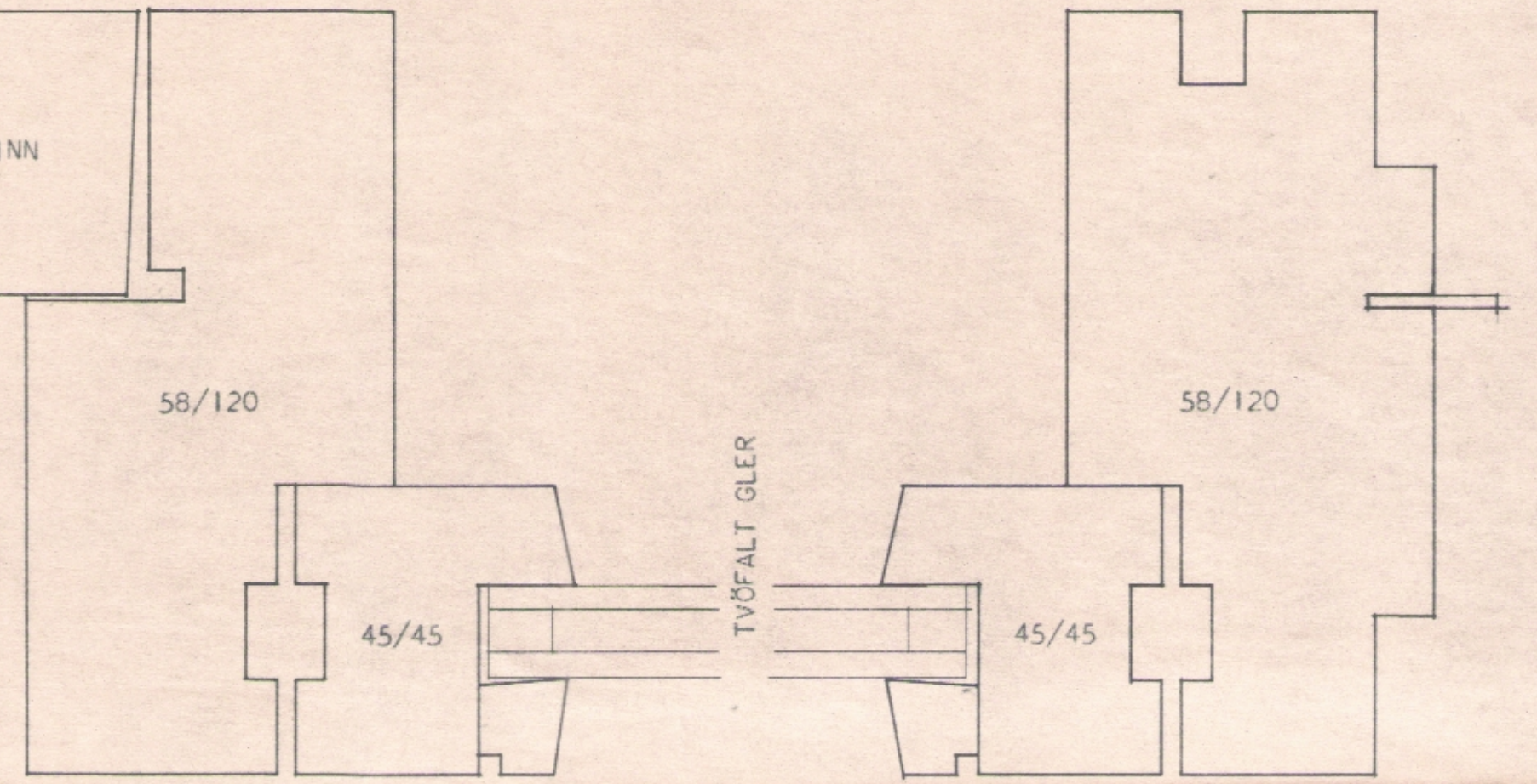
LÓDRÉTTUR PÓSTUR MILLI HURÐAR OG OPNANLEGRAR GRINDAR.
