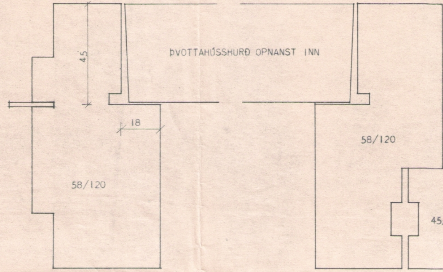
HLIDARSTYKKI MED HURÐ
