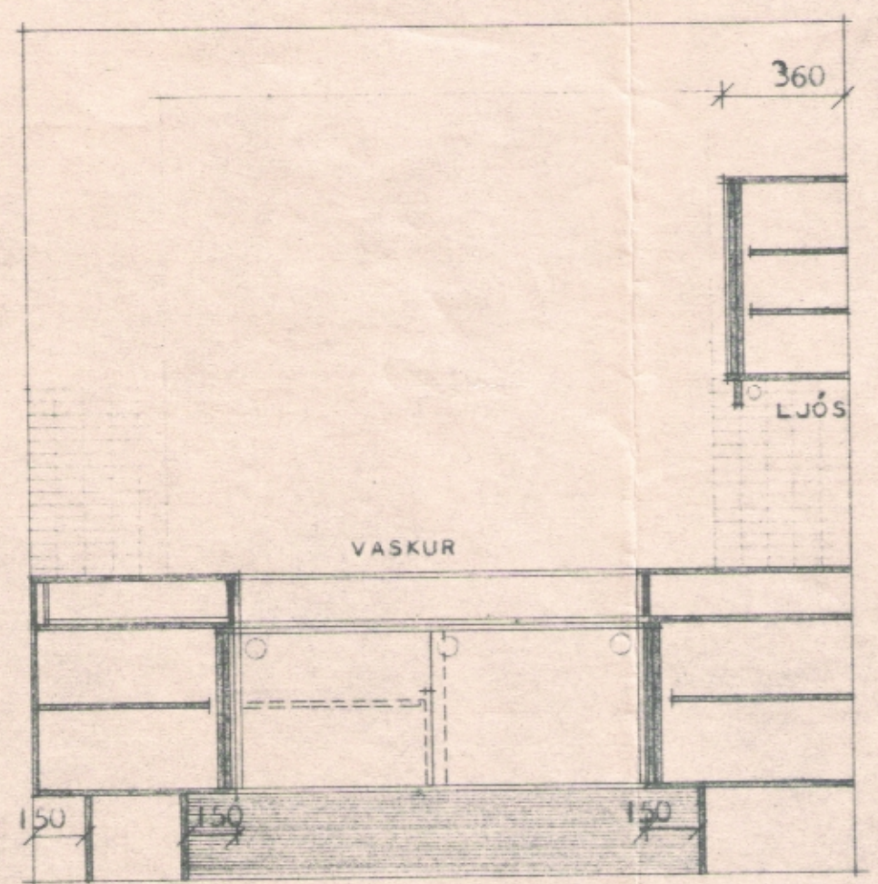
D-D
