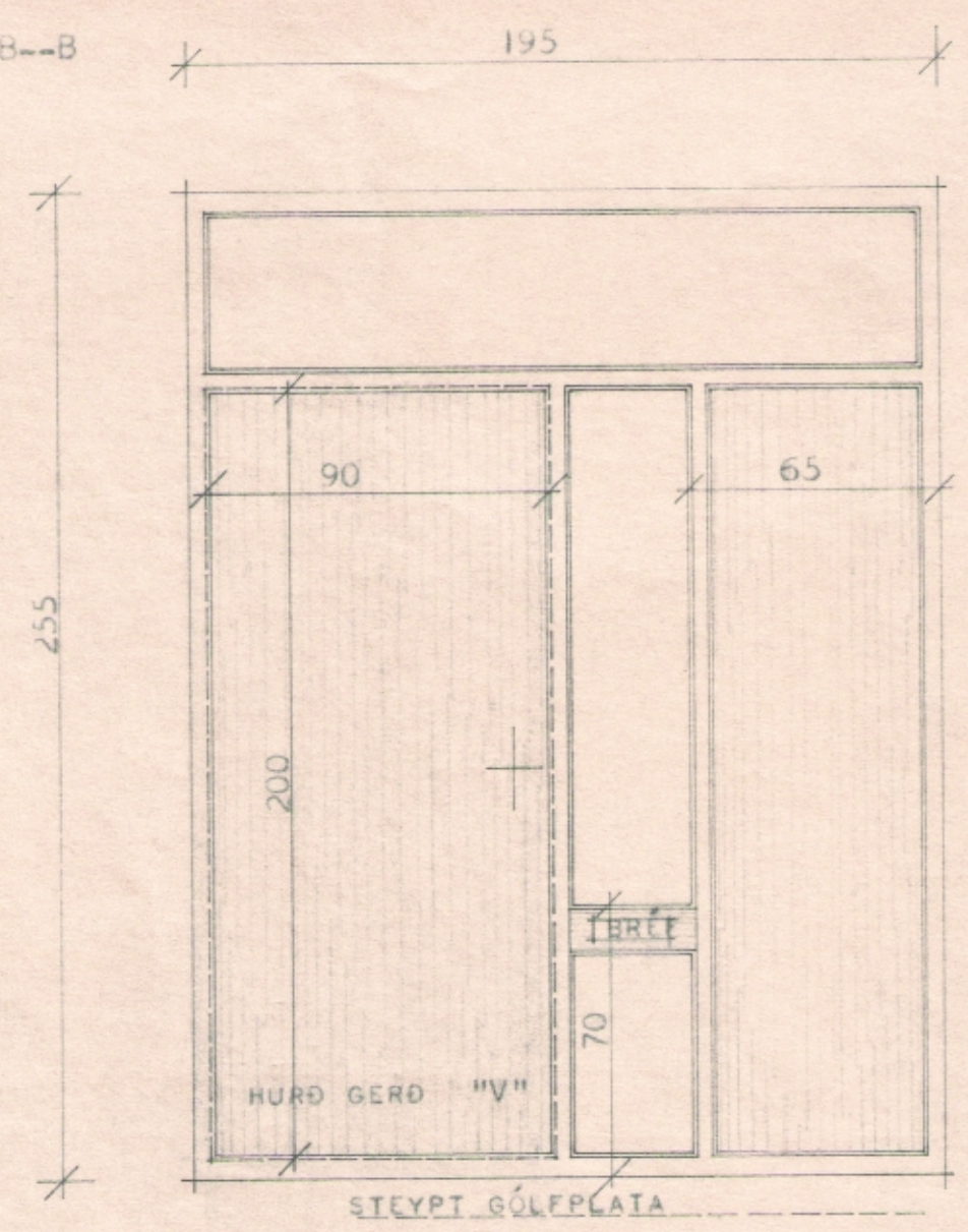
1 STK. ÚTUHURÐ. SJÁ NÁNAR BLAÐ MERKT V OG H V
