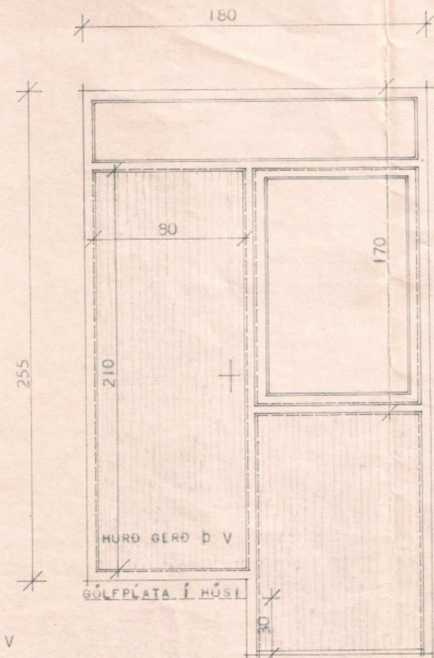
1 STK. Í ÞVOTTAHÚS. SJÁ NÁNAR BLAÐ MERKT Þ V
