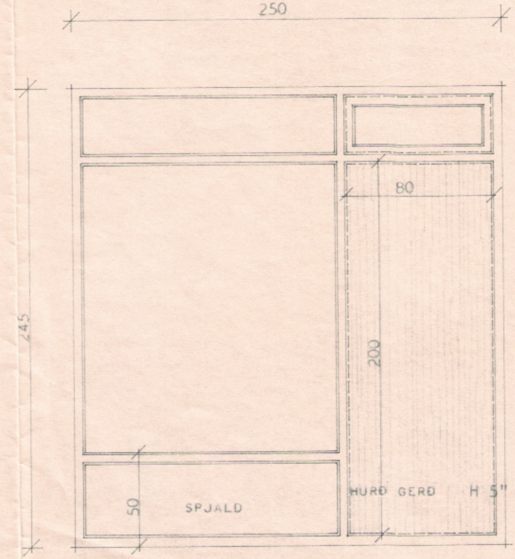
1 STK. STOFUGLUGGI. SJÁ NÁNAR BLAÐ MERKT H 5" S
