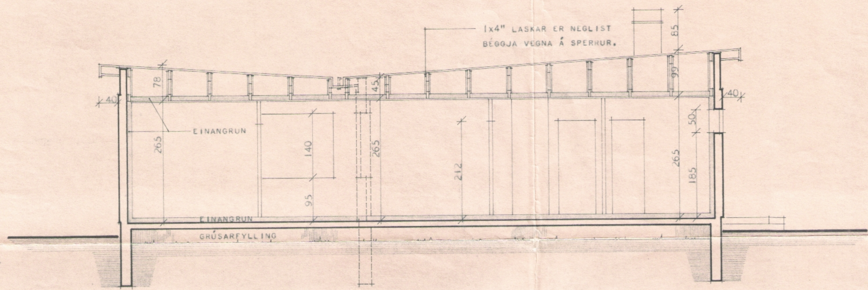
SNEIÐING A-A
