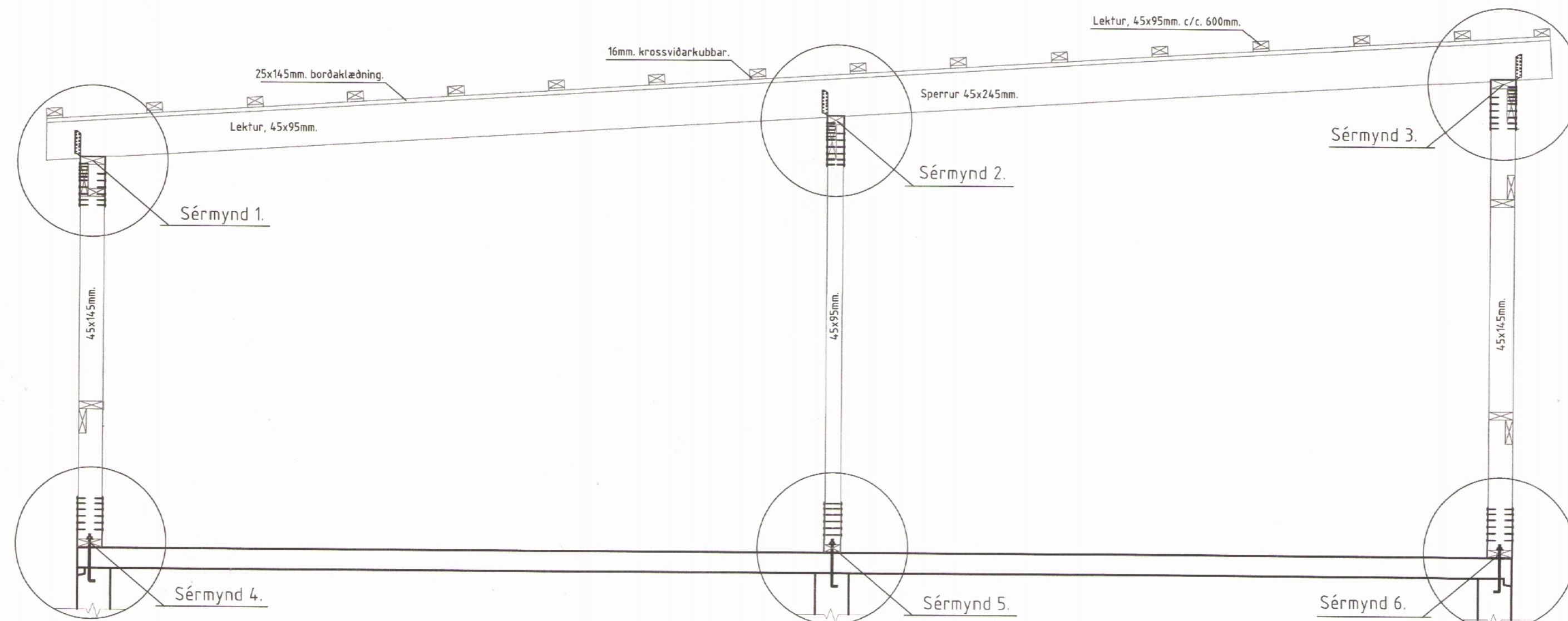
Snið A-A 1:25
