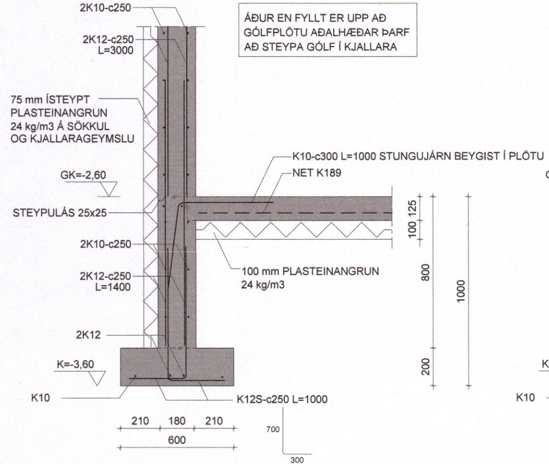
1 Snið 1:20
