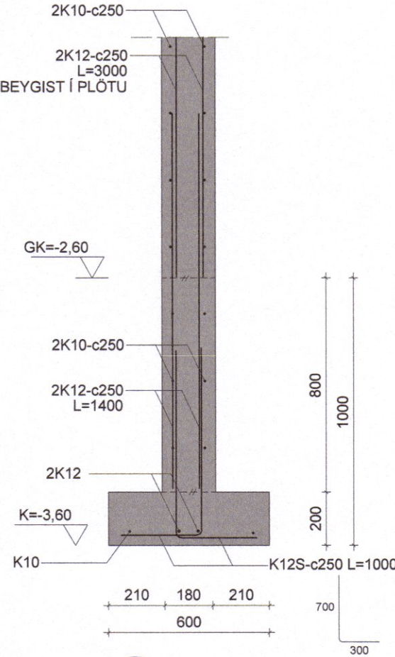
4 Snið 1:20
