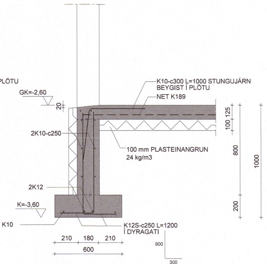
2 Snið 1:20
