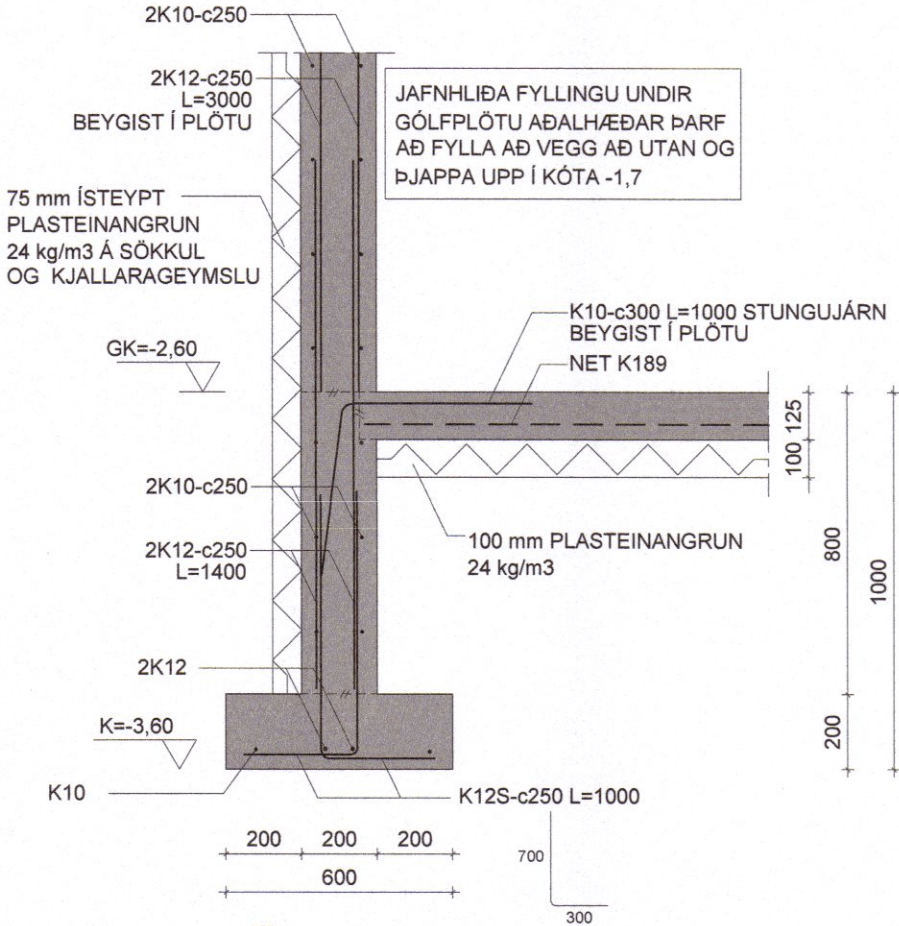
3 Snið 1:20
