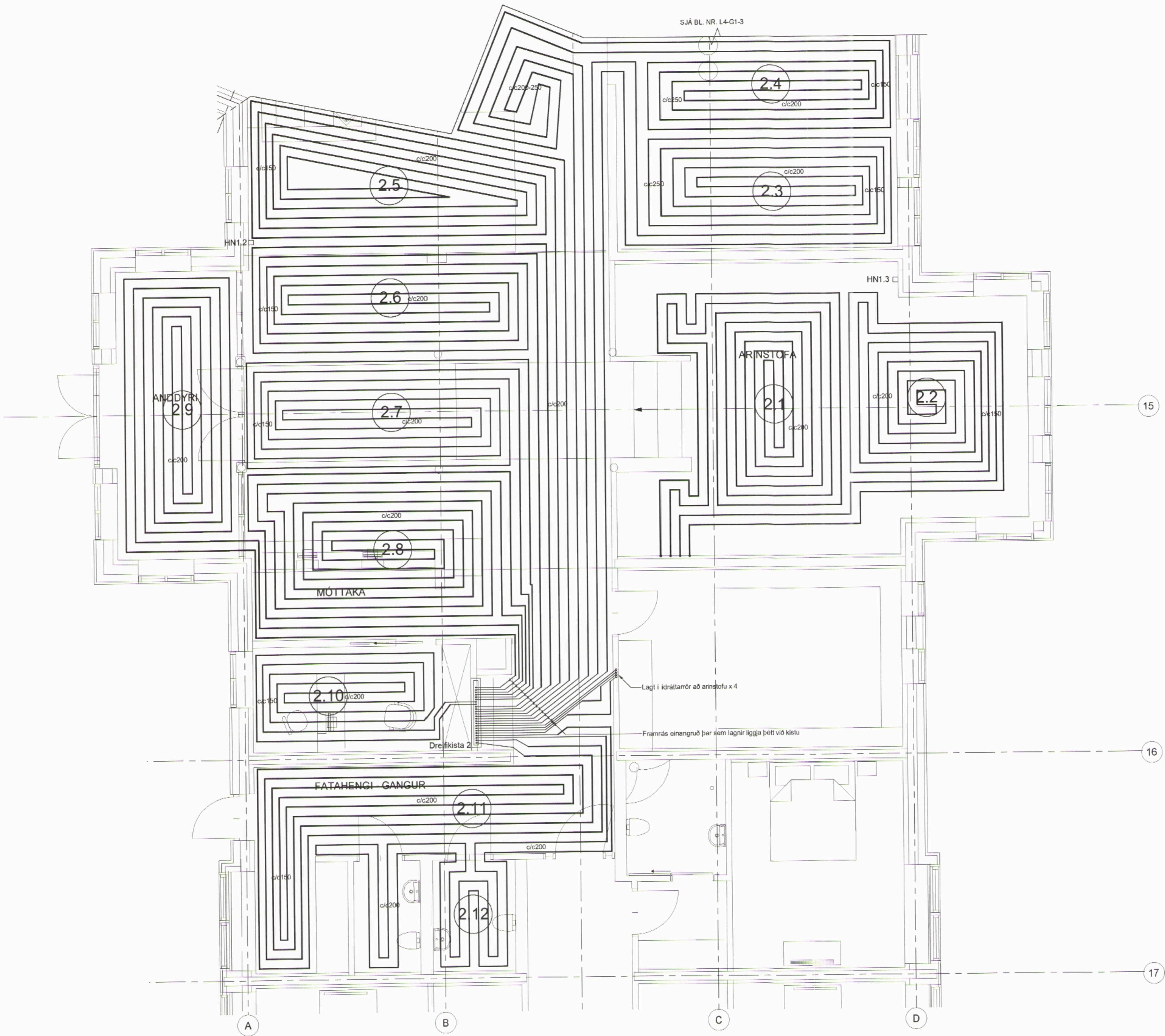
DREIFIKISTA 2 GÓLFHITASKRÁ:
