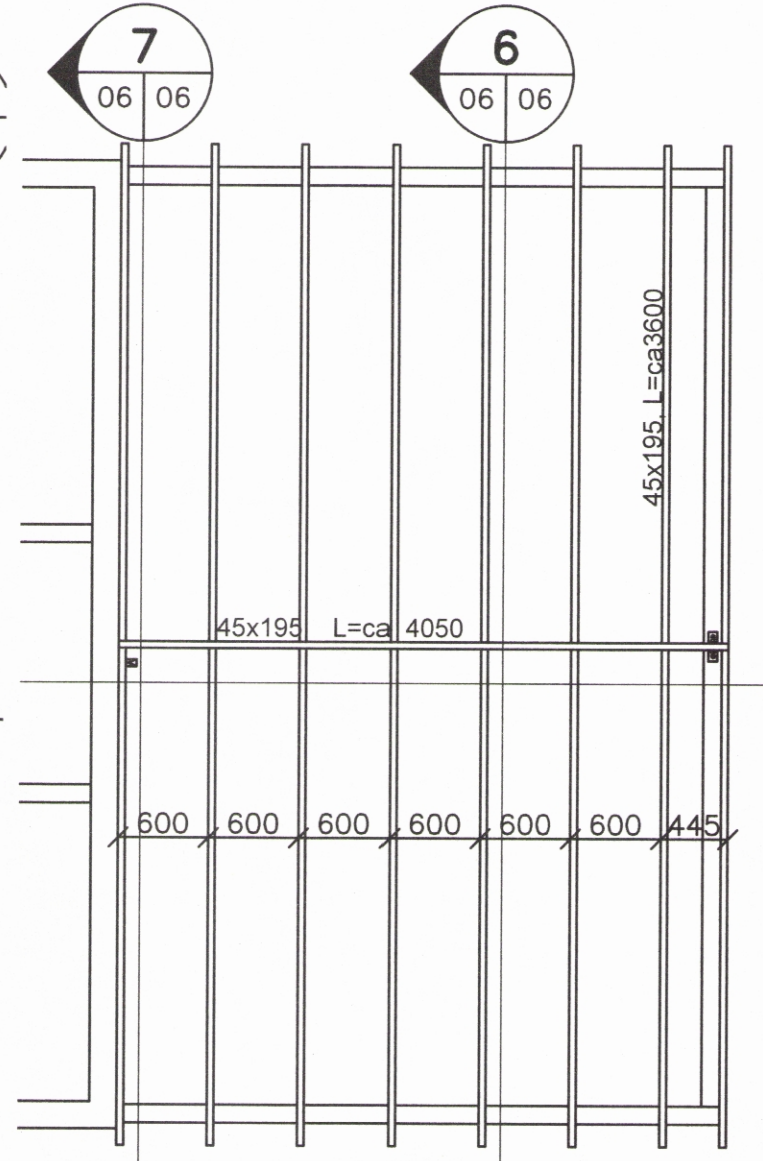
8 Þakviðir M=1: 50
