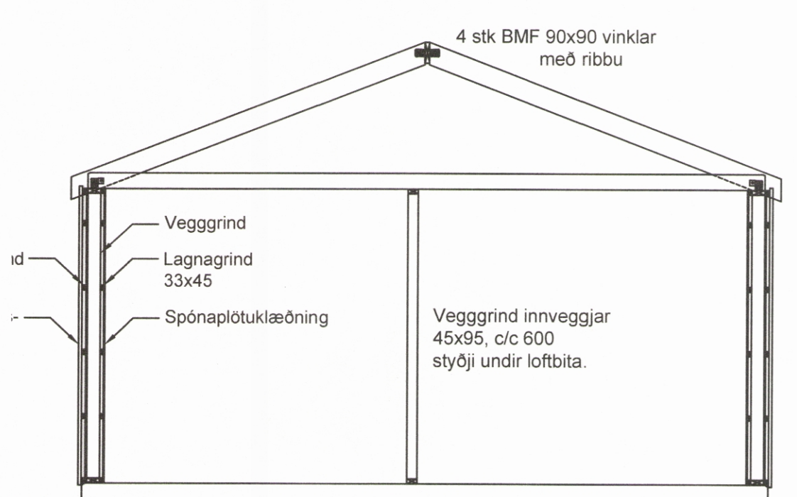
6 Snið M=1: 50
