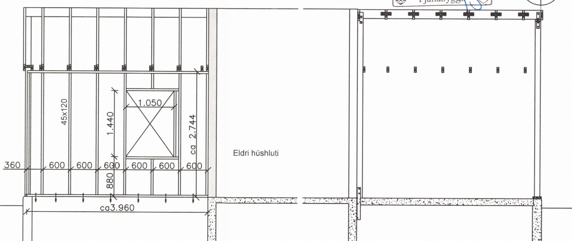
3 Vegggrind vesturveggjar M=1: 50
