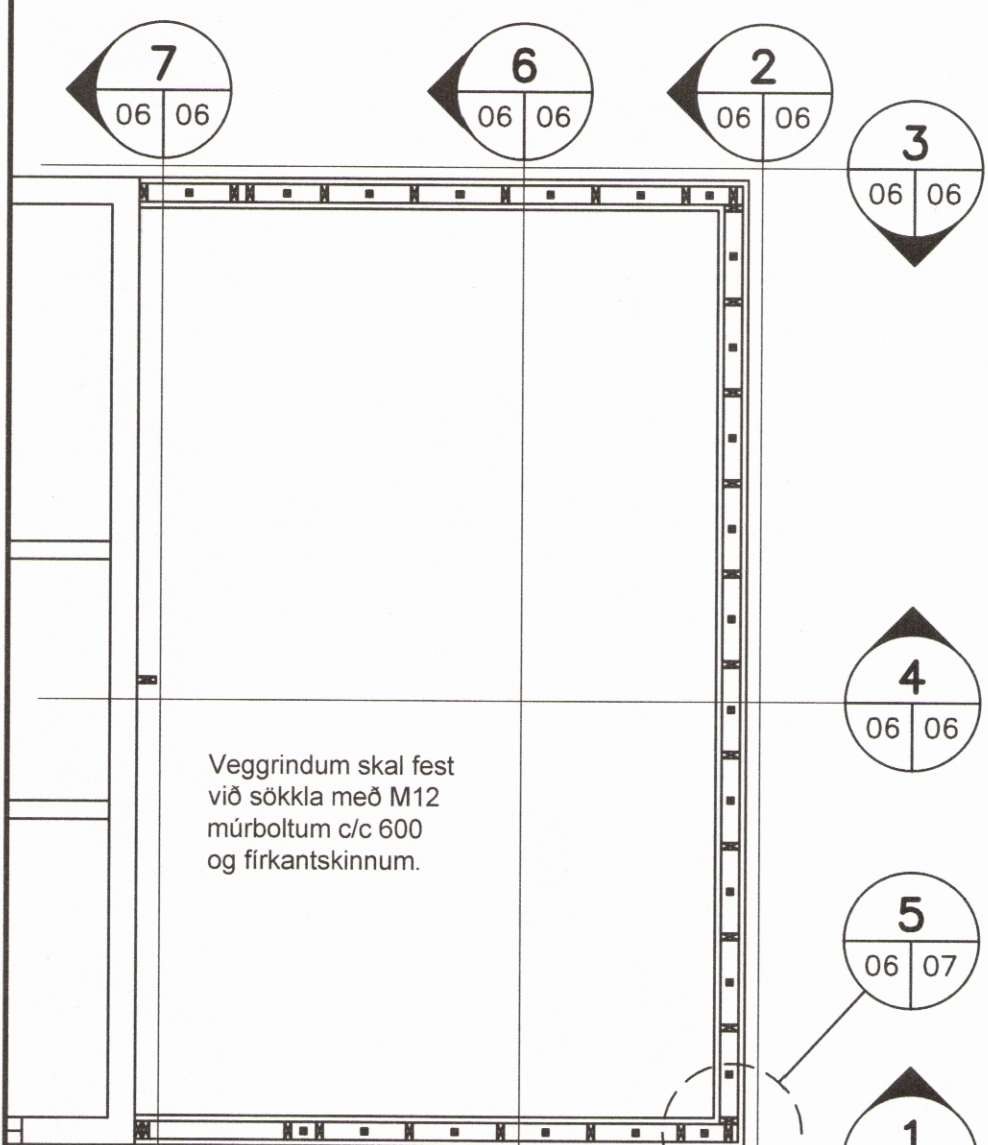
5 Grunnmynd M=1: 50
