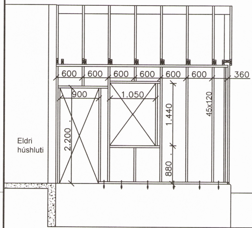
1 Vegggrind austurveggjar M=1: 50
