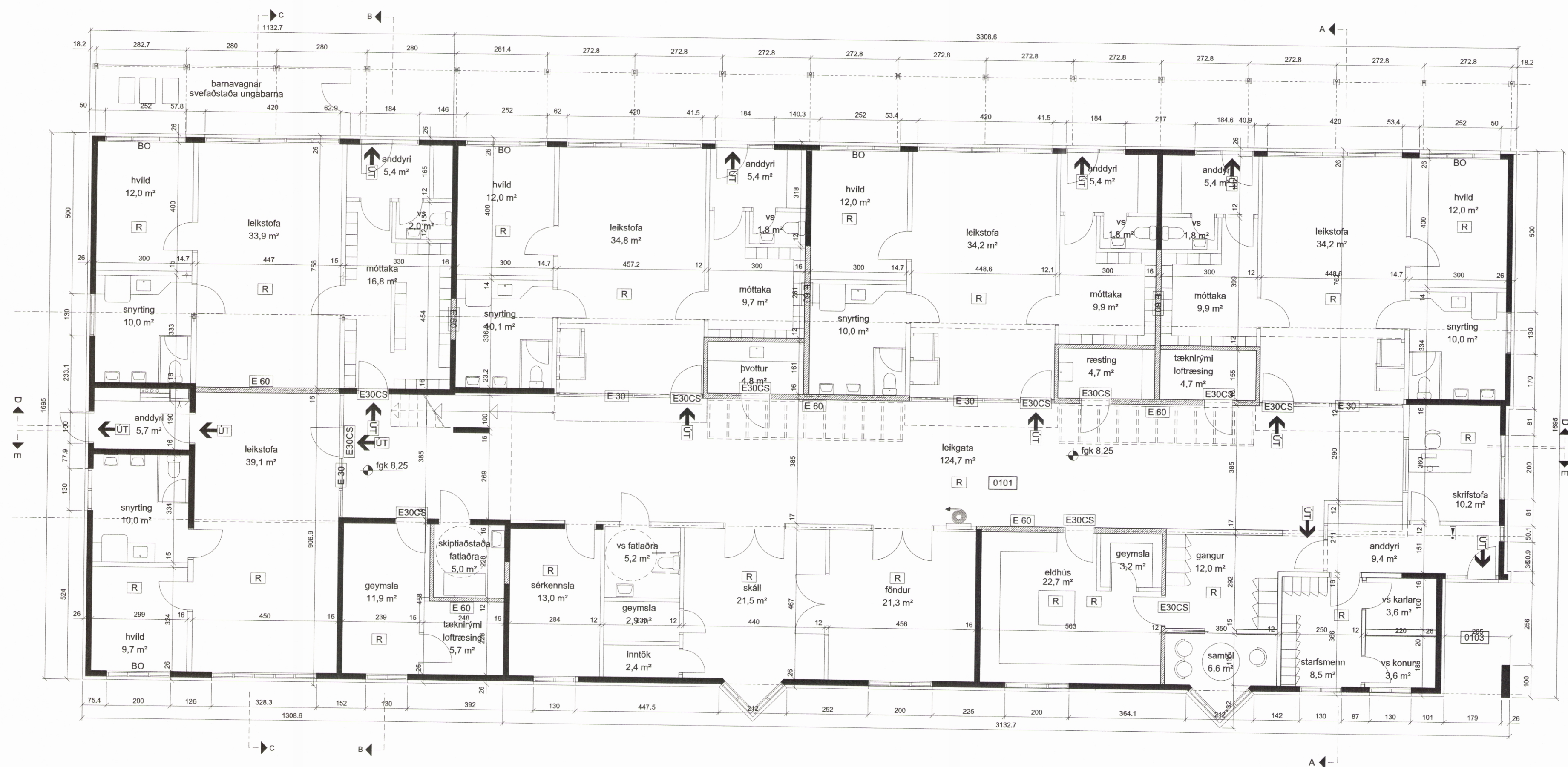
GRUNNMYND 1. HÆÐAR
