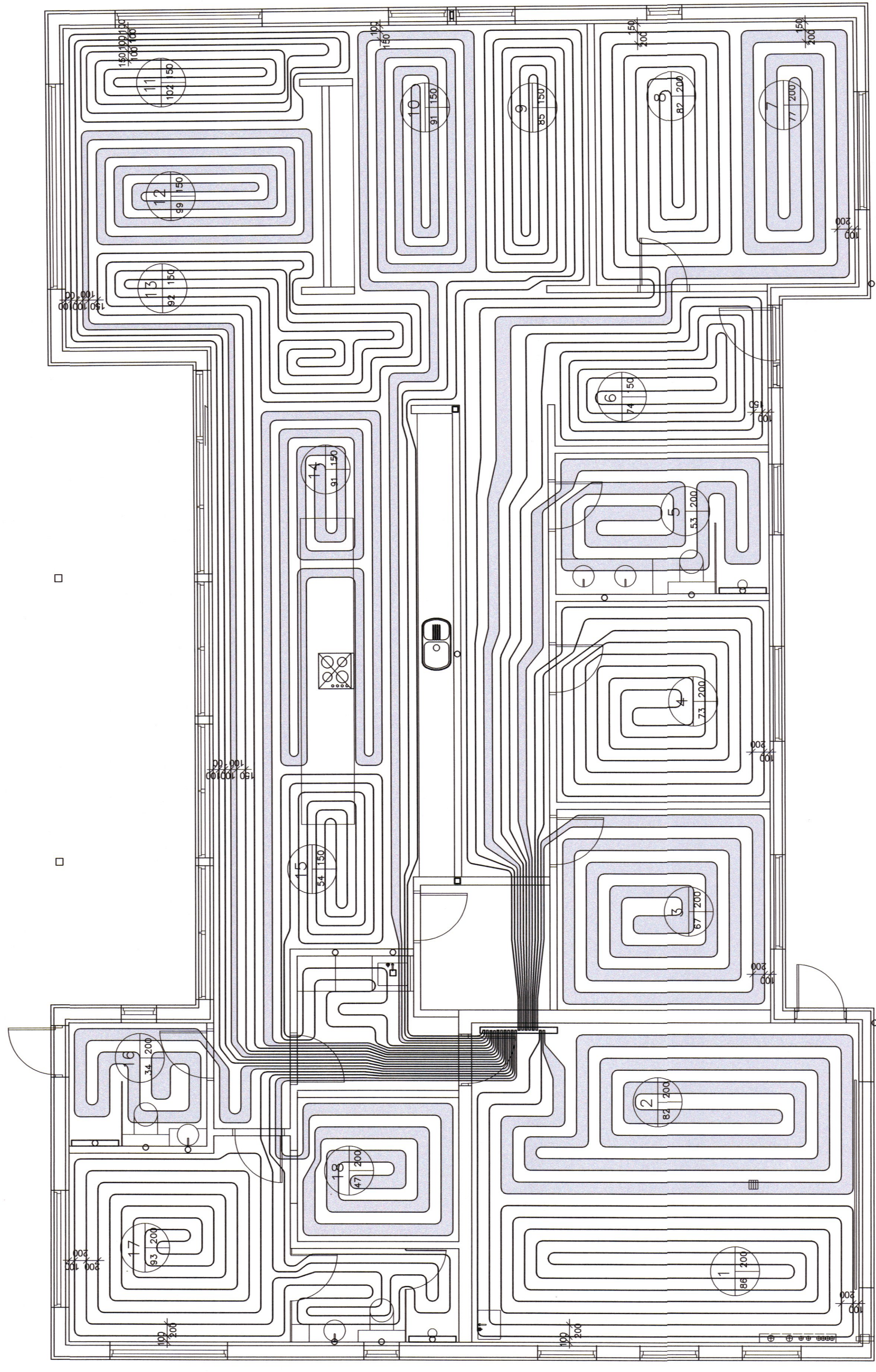
GÓLFHITALAGNIR 1:50
