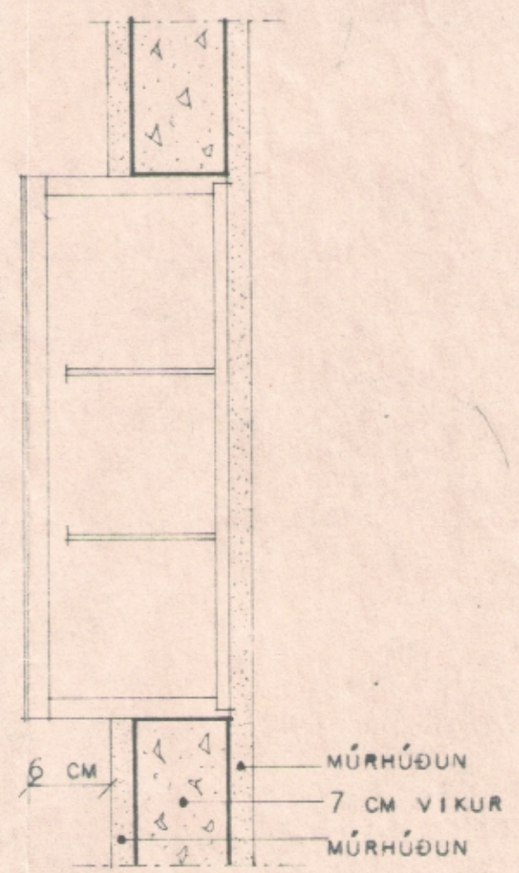
B-B
