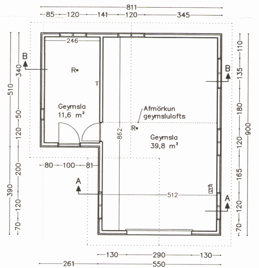
Grunnmynd 1:100
